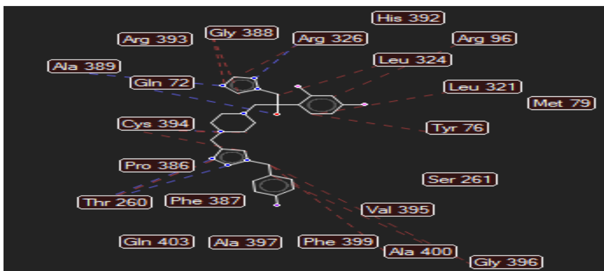
شکل ۴- بررسی رزیدوهای (آمینواسیدهای) درگیر در تشکیل پیوند مهارکننده با ترکیب شماره ۵ توسط نرم افزار مولکرو (MVD): همان‌طور که در شکل مشخص است این ترکیب با آمینواسید \text{Thr}260 ، \text{Gln}72 ، \text{Arg}326 ، \text{Ala}389 ، پیوند هیدروژنی (خط چین آبی‌رنگ) و با آمینواسیدهای \text{Leu}321 ، \text{Leu}324 ، \text{Tyr}76 ، \text{Val}395 ، \text{Ala}400 ، \text{Arg}326 ، \text{Gly}396 ، \text{Gly}388 ، \text{Cys}394 ، \text{Tyr}76 ، \text{Phe}387 ، \text{Thr}260 ، \text{Pro}386 ، \text{Phe}399 ، \text{Ala}397 ، \text{Gln}403 ، \text{Ala}389 ، \text{Arg}393 ، \text{Gln}72 ، \text{Leu}321 ، \text{Met}79 ، \text{Ser}261 ، \text{Val}395 ، \text{Ala}400 ، \text{Gly}396 برهم‌کنش‌های هیدروفوبیک در تشکیل پیوند هیدروفوبی (خط چین قرمز رنگ) شرکت می‌کند.
