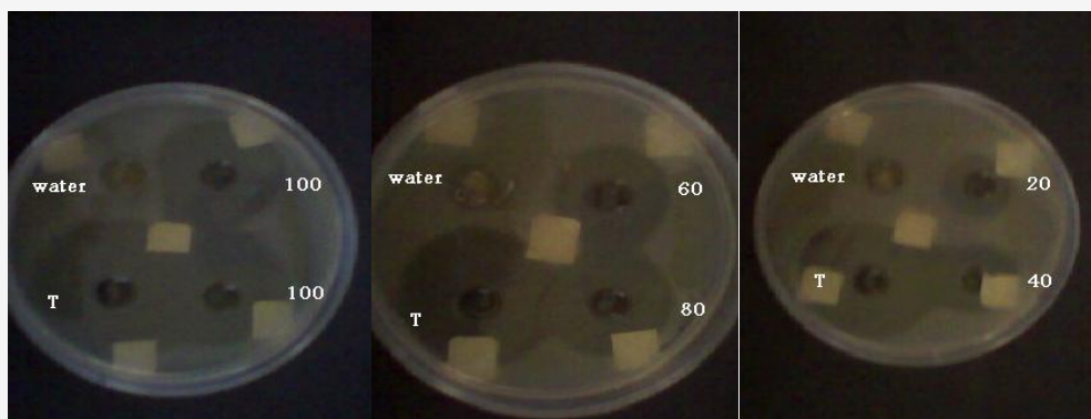
شکل ۳: نواحی بازداري باکتری آئروموناس هیدروفیلا در غلظت‌های مختلف نانو ذرات CuO
