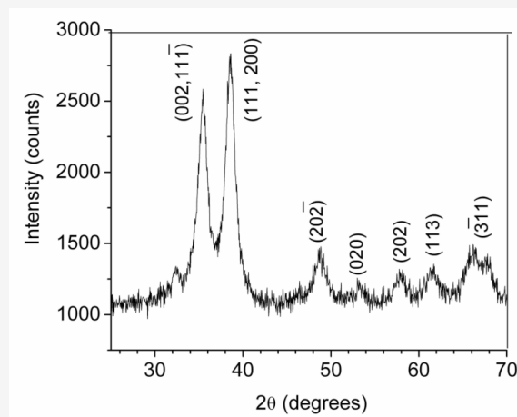
شکل ۲: طیف پراش پرتو X- (XRD) نانو ذرات CuO
