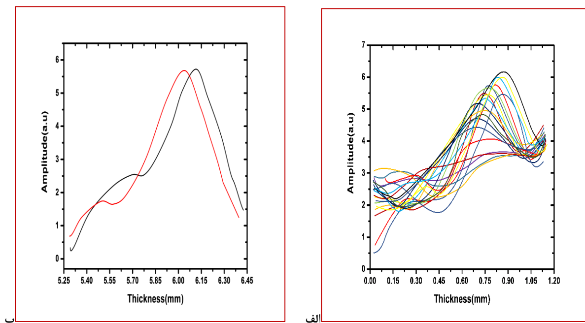
شکل ۵- تغییرات ضخامت گوه پوشش داده شده با کلسترول اولات نمایش داده شده است. (الف) جابجایی پیک متغیر (شیب‌دار گوه) نسبت به سطح ثابت (پایین گوه). (ب) دونقطه مشخص از گوه جهت نمایش تغییرات.
