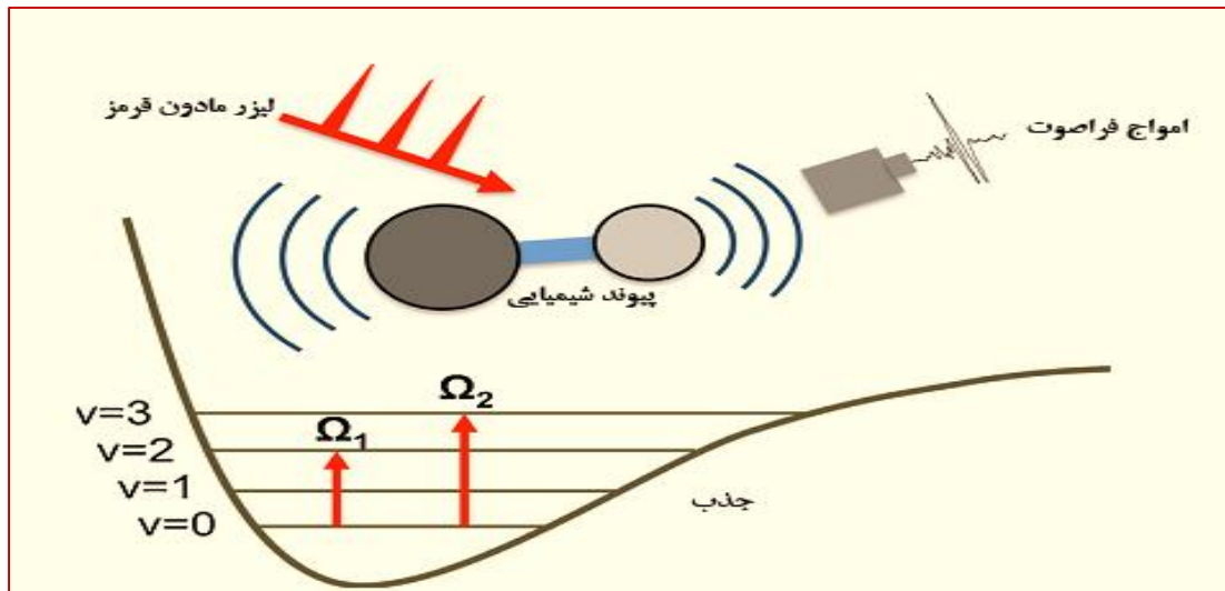
شکل ۱- نحوه تولید سیگنال فوتوآکوستیک مبتنی بر ارتعاش و جذب انرژی دریافتی در سطوح انرژی ارتعاشی اول و دوم یک مولکول (۱۴)
