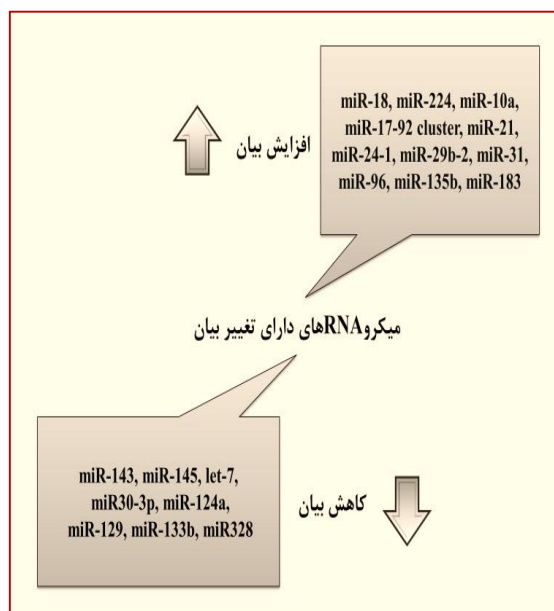
شکل ۲- برخی میکروRNAهای دارای افزایش بیان یا کاهش در سرطان کلوئید کال (۴۲)
