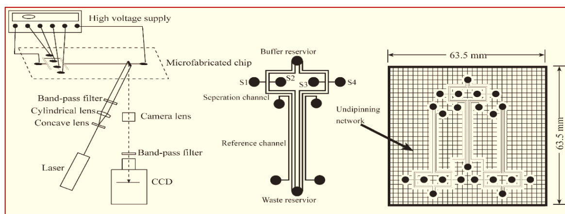
شکل ۵- شماتیک دستگاه و تراشه‌ی الکتروفورز موین ساخته شده توسط شن و همکاران (۳۹)
